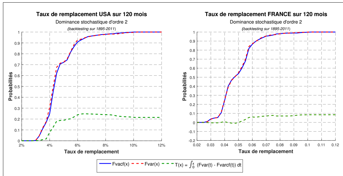
FIGURE 2.33 – Taux de remplacement & Dominance stochastique pour 120 mois
