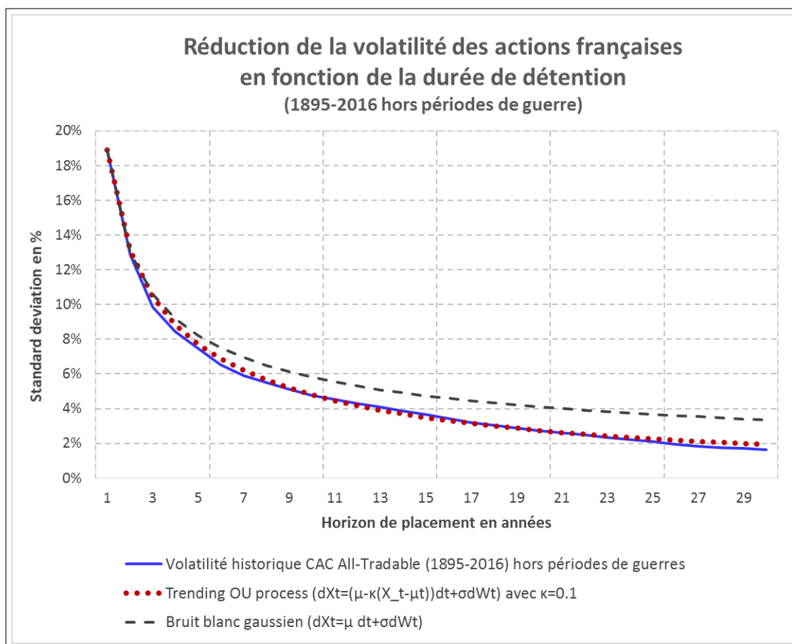
FIGURE 5.17 – Reduction de la volatilité - Actions françaises
