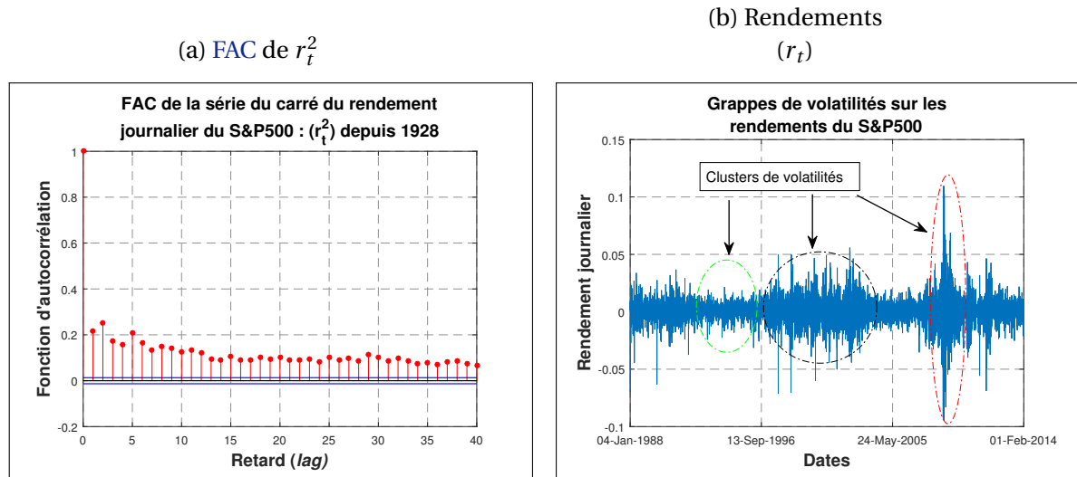
FIGURE 3.1 – Illustration de variance autoregressive des rendements sur le S&P500
