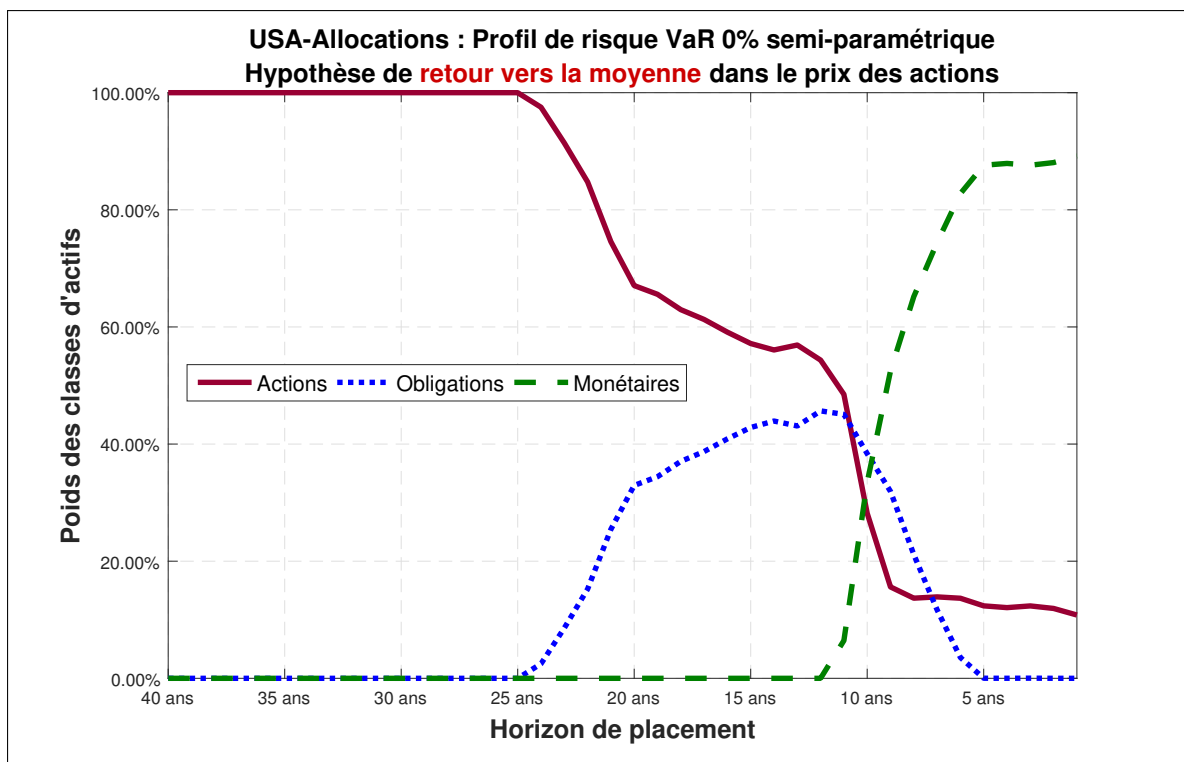
FIGURE 2.27 – USA : Allocations - VaR 0% semi-paramétrique
