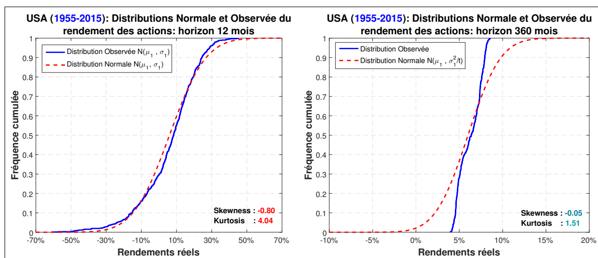
FIGURE 2.10 – Fonctions de répartition - actions américaines (1955-2015)
