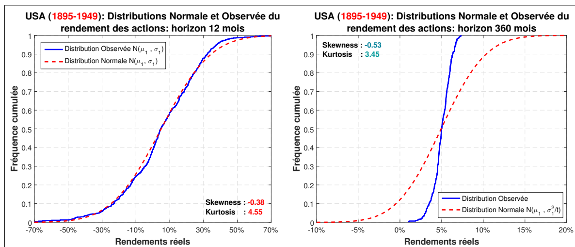
FIGURE 2.9 – Fonctions de répartition - actions américaines (1895-1949)
